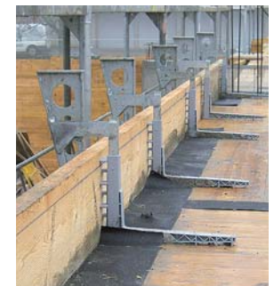
Recouplement latéral
